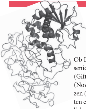
Bändermodell des Rizins nach PDB Zaal. Dunkel die A-Kette, hell die B-Kette dargestellt.
